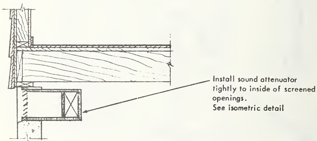
b - Vent attenuators
