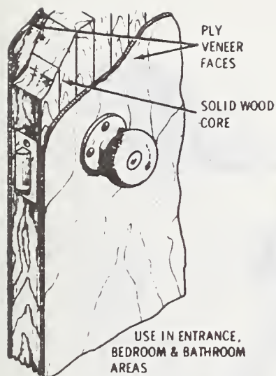
SOLID CORE DOOR
