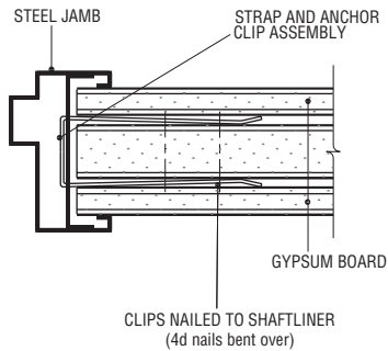
JAMB DETAIL 09250X Scale: 3" = 1'-0"
