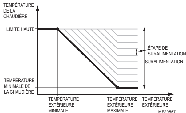
Fig. 3. La courbe de compensation de température extérieure avec suralimentation.
