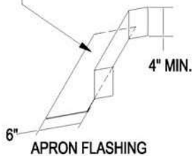
APRON FLASHING
