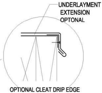
OPTIONAL CLEAT DRIP EDGE
