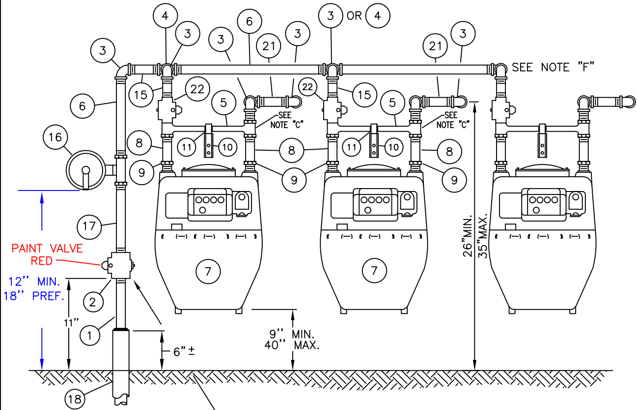
ELEVATION
