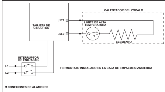
Cableado de la Caja de Empalmes - Izquierda
