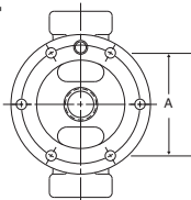
Fig. 27-1. Bolt Circle
